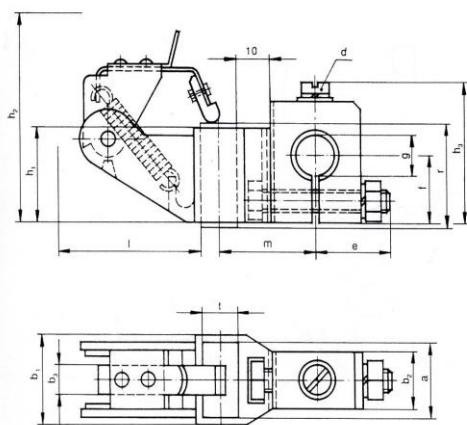
mit Klemmstück K
