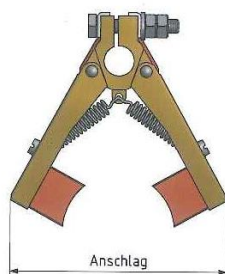
G/A (ohne Winkel, mit Anschlag)
